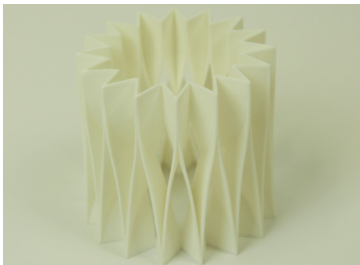
Abb. 9 3D (PLA) Filamentdruck zu Gefaltetem Stützelement.
